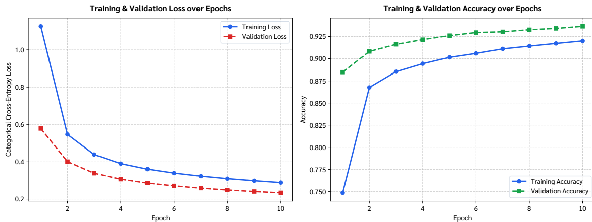
รูปที่ 3: Learning Curves for Baseline DNN (Mini-batch SGD, lr=0.01, Batch=128): ซ้าย: ค่า Categorical Cross-Entropy Loss บนชุด Train และ Validation ขวา: ค่า Accuracy ตลอด 10 Epochs
